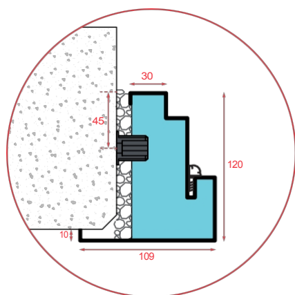
DØRKARM - DSA B IM
