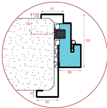
DØRKARM B MED UNDERKARME
