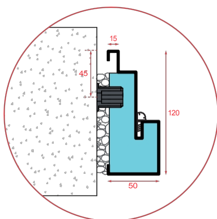
DØRKARM - DSA C15
