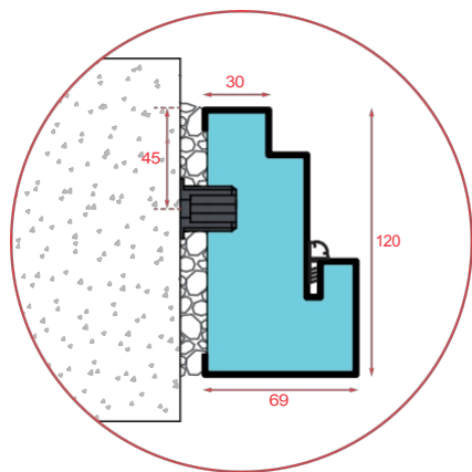
DØRKARM - DSA C
