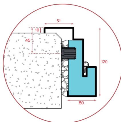
DØRKARM - B
